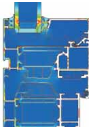
Schüco SelectLine Innovative Technik sorgt für optimale Wärmedämmung
