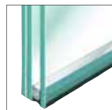
Aufpreis: Einbruchhemmendes Glas SchücoTherm Ultra 1.1 A3 Glasaufbau A3 (9)-16-4 mm U_g: 1,1 \text{ W/m}^2\text{K} R_w: 38 \text{ dB}
